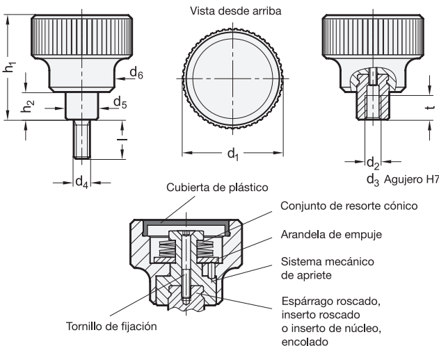
GN 3663-con perno roscado
